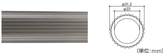
積水樹脂 内窓・縦長手すり兼用 パイプ
