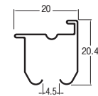
レール断面図(単位:mm)
