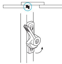
3枚引違いの取付例 (向かって左側の窓が手前にある場合)
