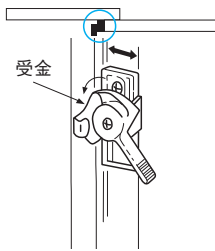
2枚引違いの取付例
